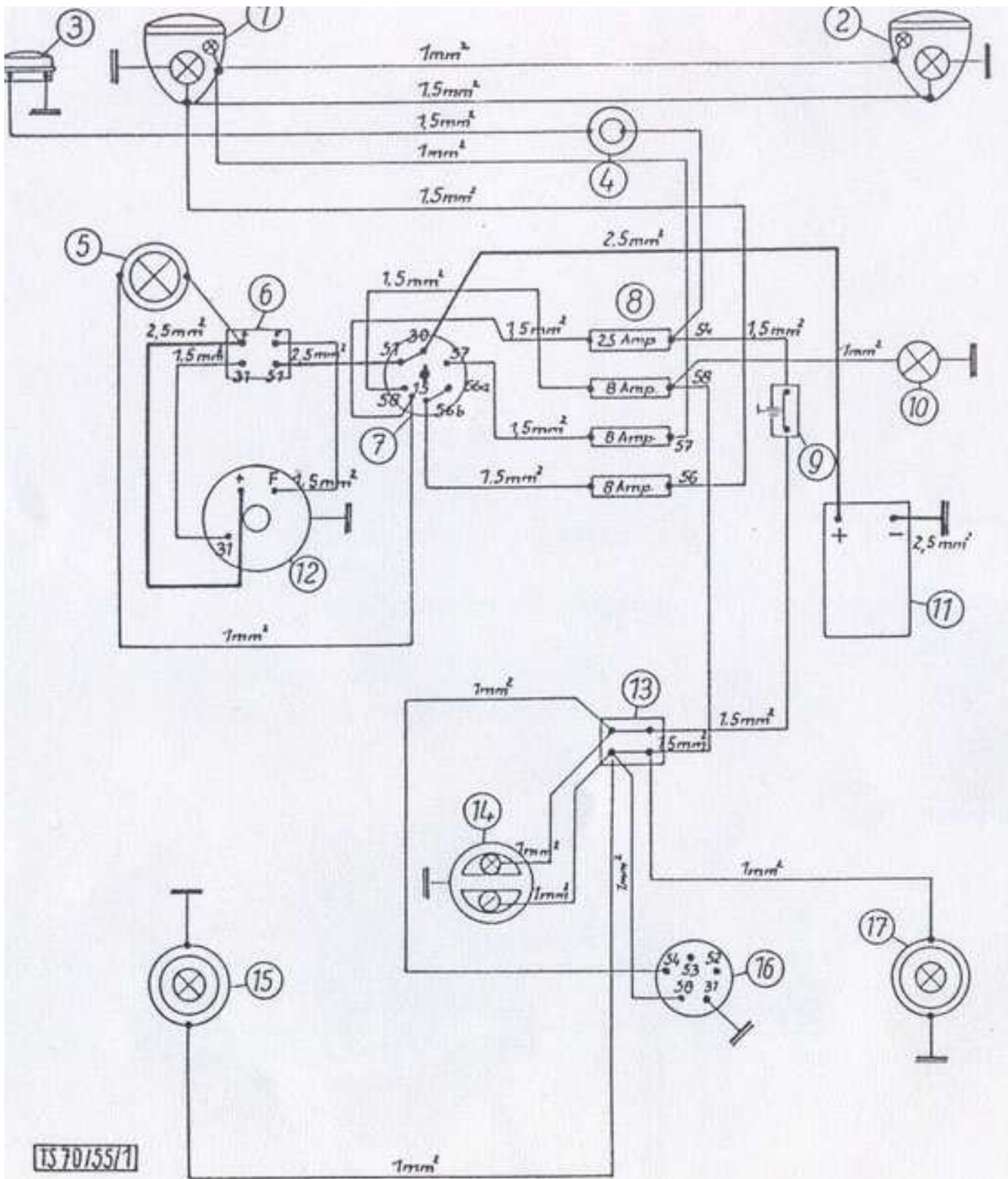
Bild 28: Elektrischer Schaltplan 6-Volt-Anlage
